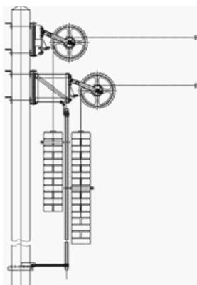
شکل (۳-۹) کشش جداگانه سیم‌های حمال و کنتاکت
