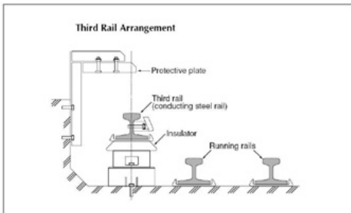
شکل (۳-۱۳) ساختار ریل سوم
