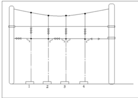
شکل (۳-۱۲) Suspension head span
