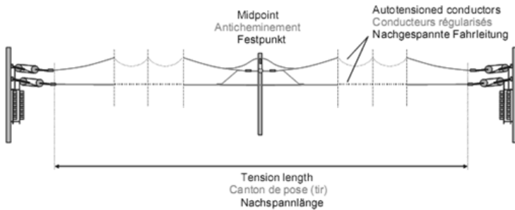
شکل (۸-۳) یک section شبکه OCS
